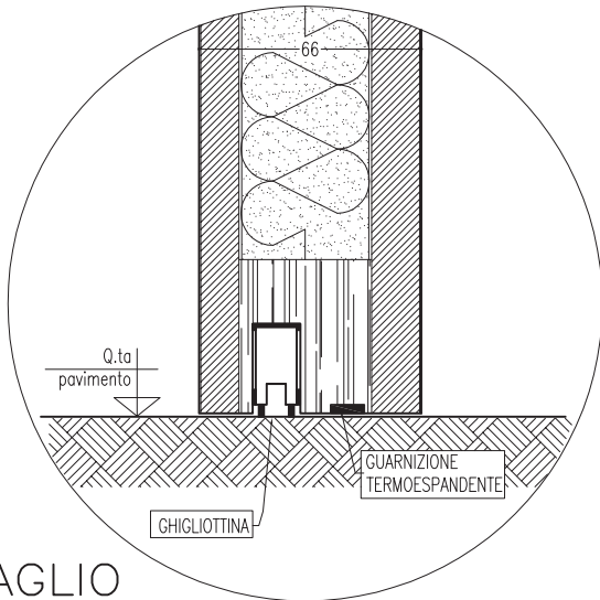
SEZIONE VERTICALE
