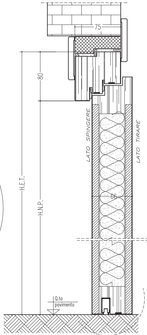
SEZIONE VERTICALE
