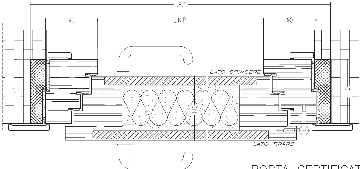
SEZIONE ORIZZONTALE
