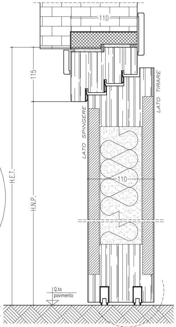
SEZIONE VERTICALE
