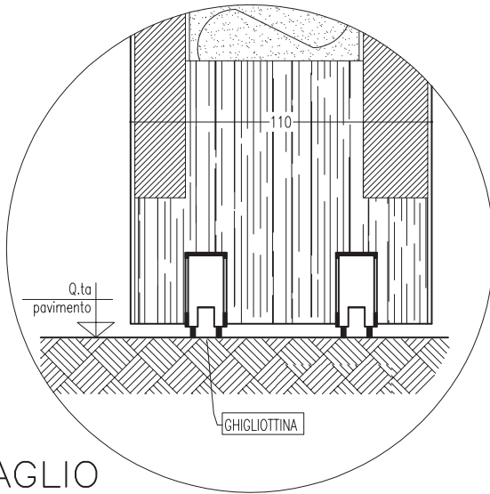
SEZIONE VERTICALE
