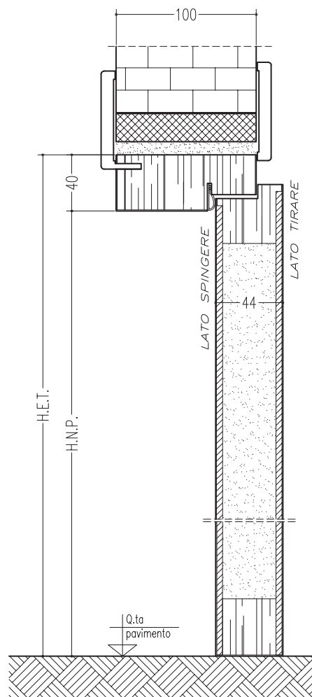
SEZIONE VERTICALE
