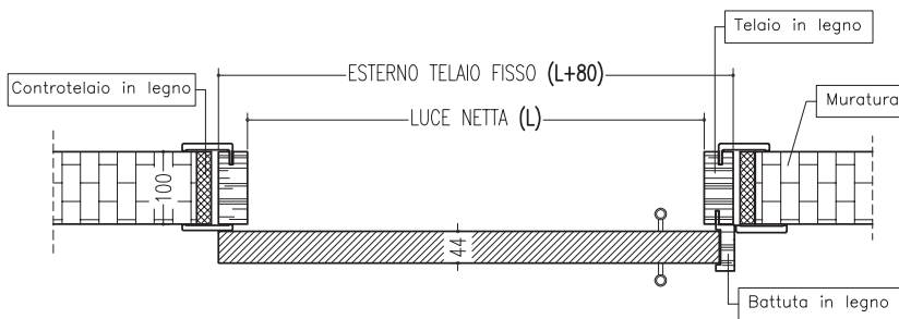
SEZIONE ORIZZONTALE
