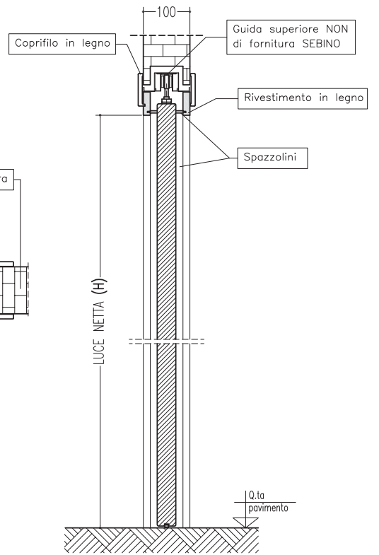
SEZIONE VERTICALE
