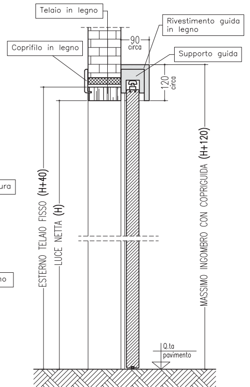
SEZIONE VERTICALE
