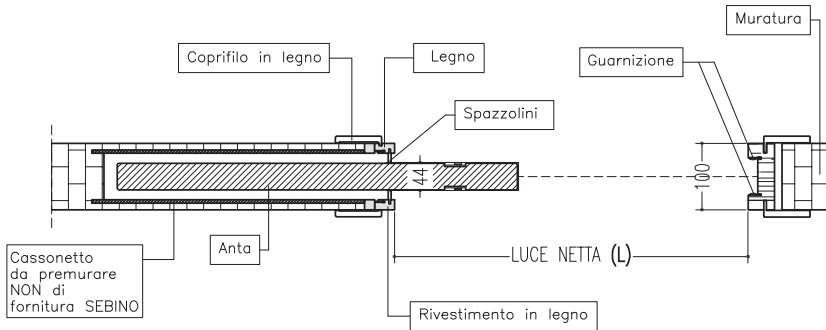
SEZIONE ORIZZONTALE
